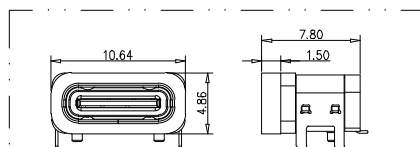
加防水圈示意图
