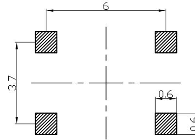
安装参考图
